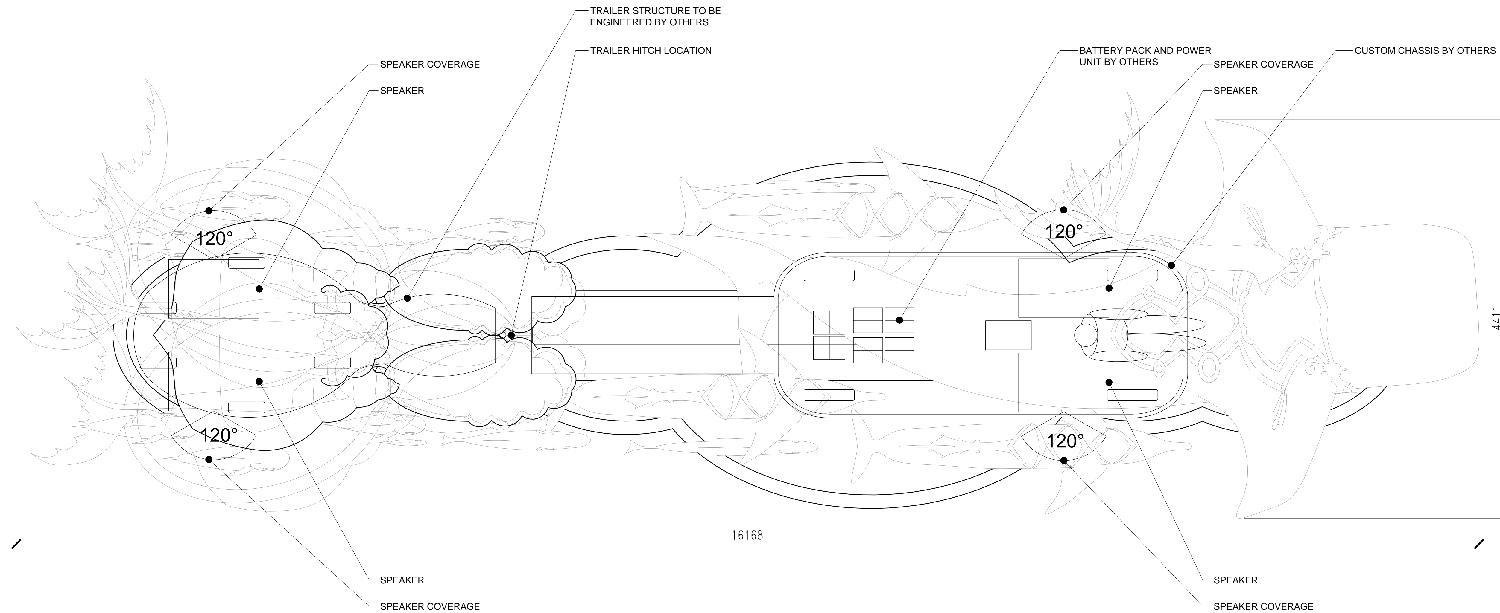
4 CHIMELONG PARADE FANFARE PLAN 1:25
